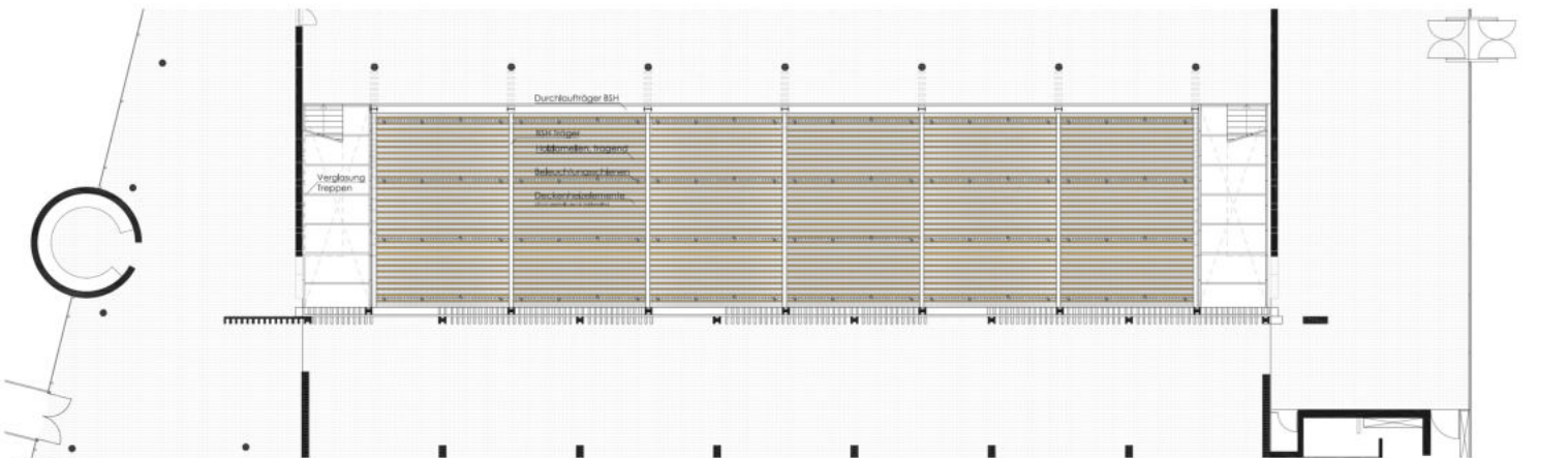
DECKENSPEZIEL M:1/100
