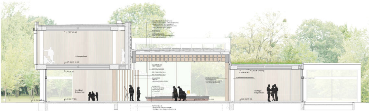
DETAILSCHNITT M:1/50
